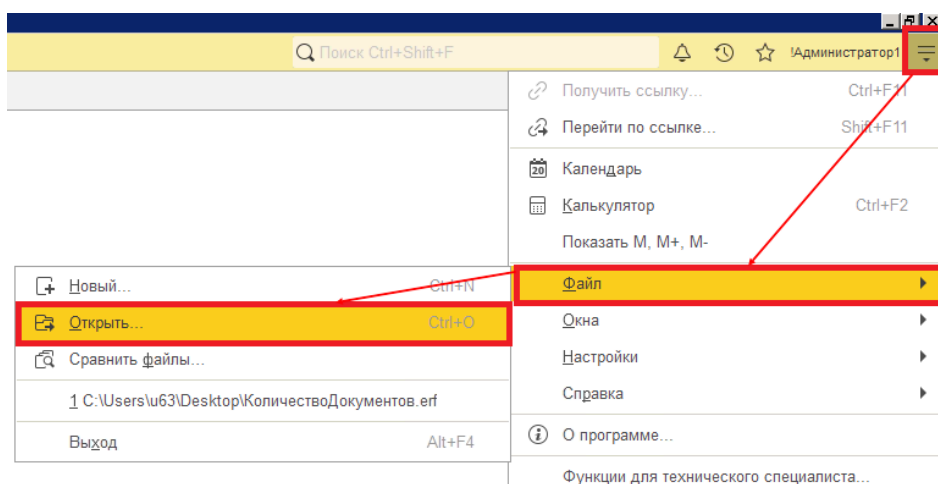
Рисунок 1. Схематическая последовательность действий для вызова диалогового окна открытия внешнего отчета
